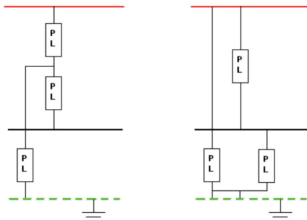
Figura 8 – Exemples de connexió dels dispositius parallamps.
