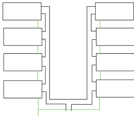
Figura 11 – Exemple d'embrancament correcte: reducció de les superfícies dels cables.
