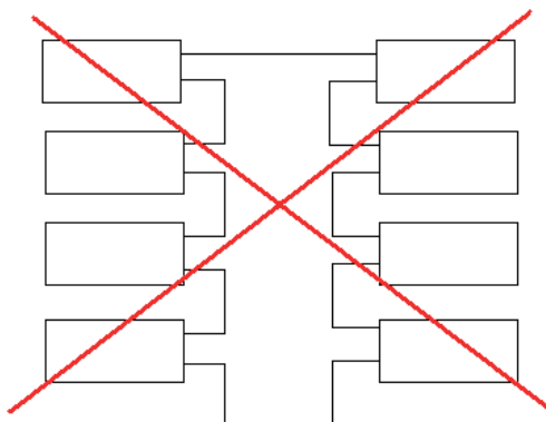
Figura 9 – Exemple d'embrancament incorrecte: inducció entre polaritats.
