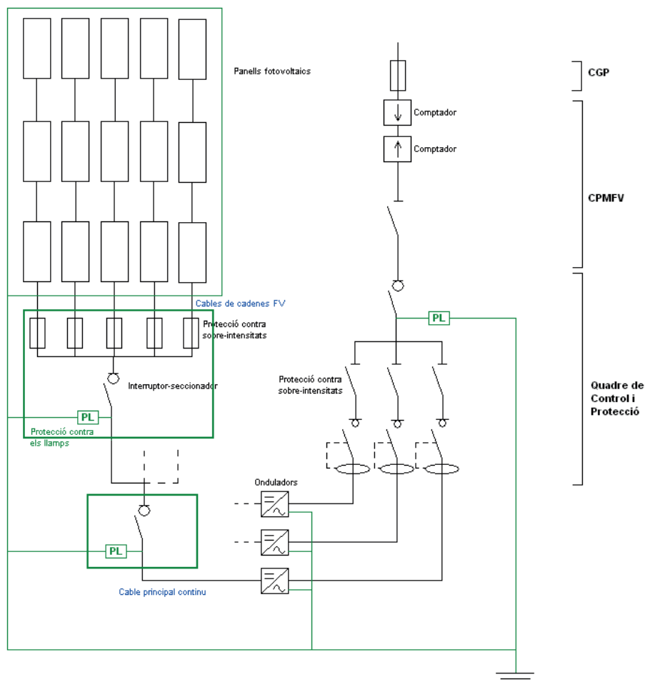
Figura 2 – Esquema de principi d'una instal·lació fotovoltaica.
