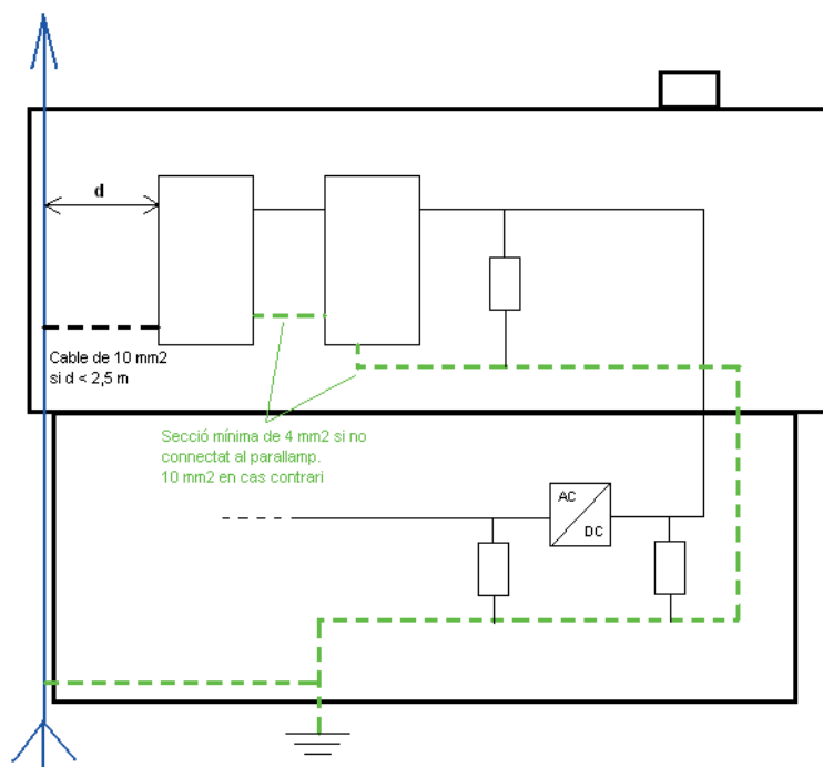
Figura 3 – Exemple d'instal·lació amb protecció per punta parallamps.
