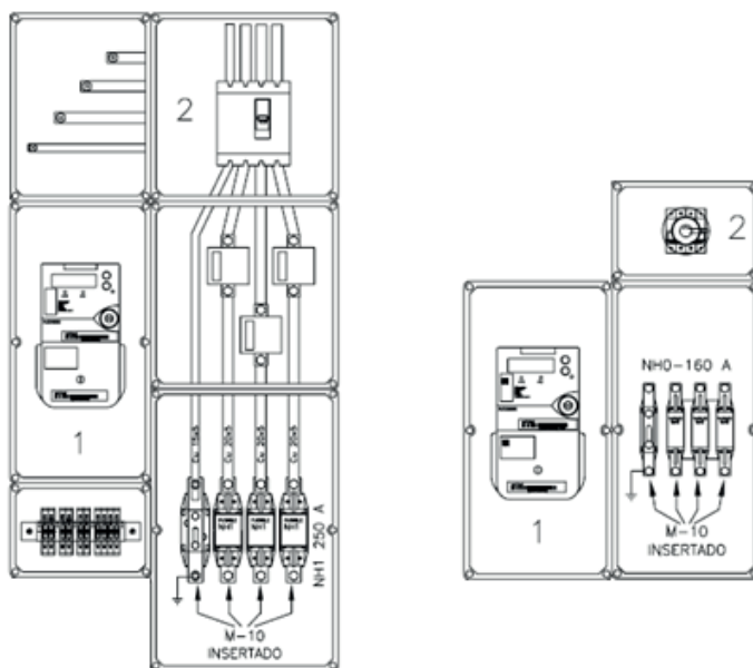
Figura 6: Exemples de CPMFV
