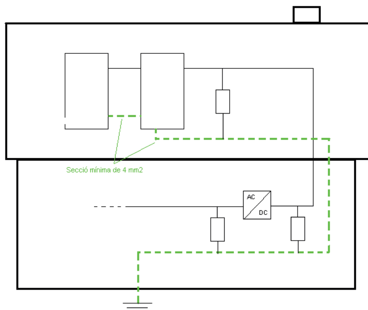
Figura 4 – Exemple d'instal·lació sense protecció per punta parallamps.
