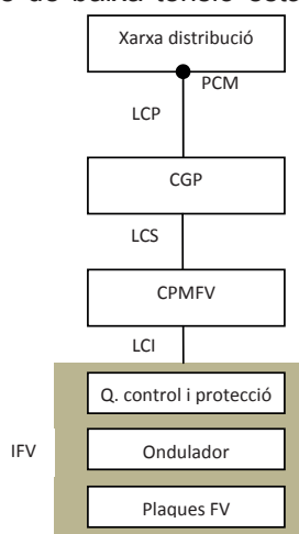
Figura 1: Esquema de blocs
