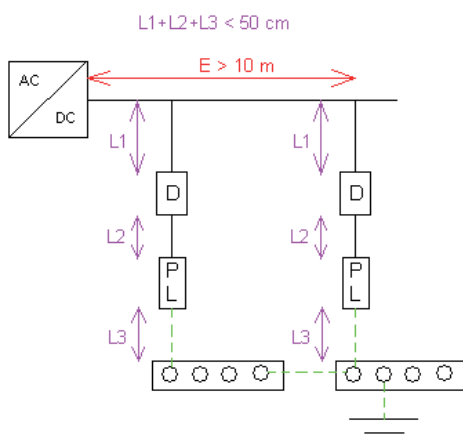
Figura 6 – Distància E > 10 metres.
