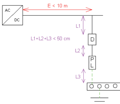
Figura 5 – Distància E < 10 metres.
