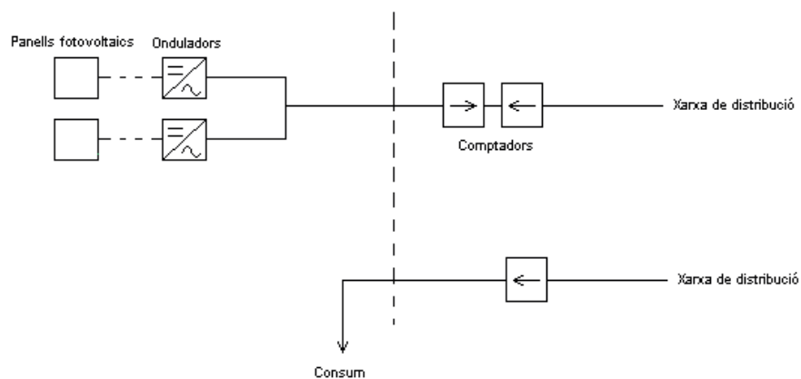
Figura 1 – Embranchament a la xarxa en dos punts.
