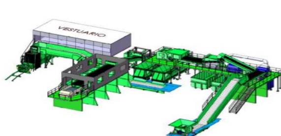
Figura 39. Maquinària de la planta i bales de materials plàstics resultants de la classificació al CTE
