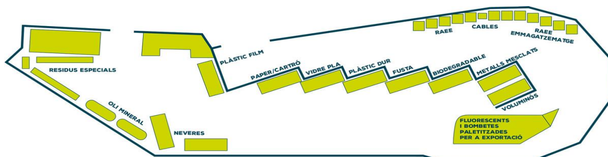
Figura 9. Distribució dels contenidors per dipositar els diferents residus a la deixalleria industrial del CTR
