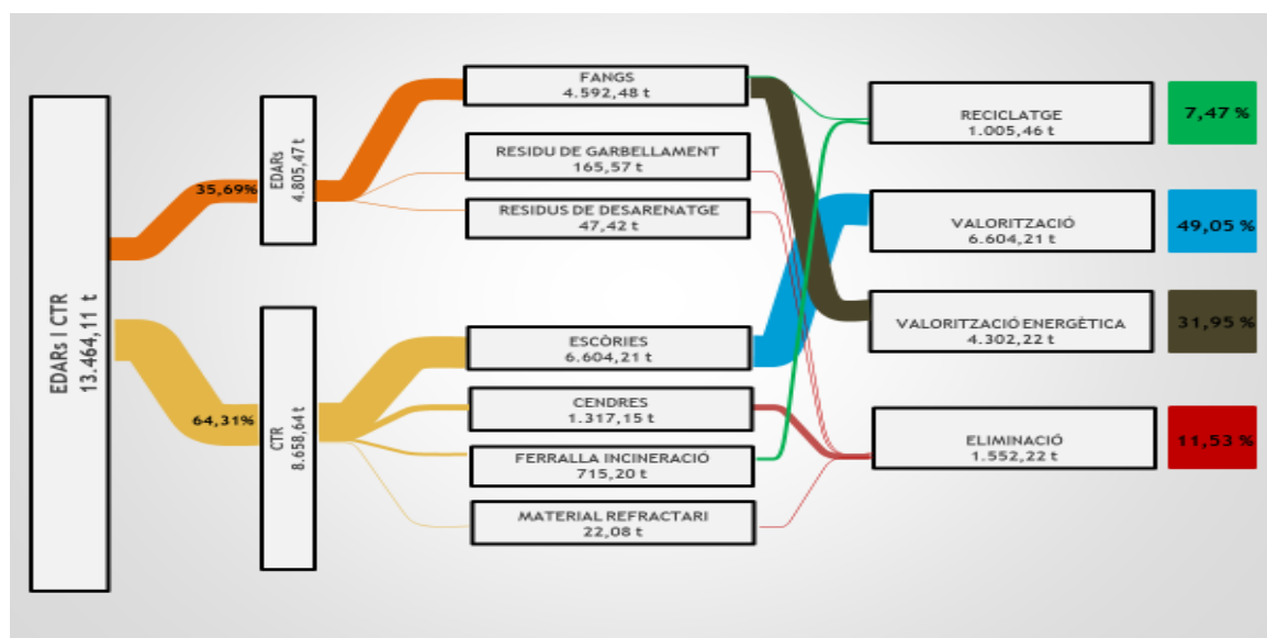
Figura 7. Flux de residus per al sector de les EDAR i CTR per al 2019.
